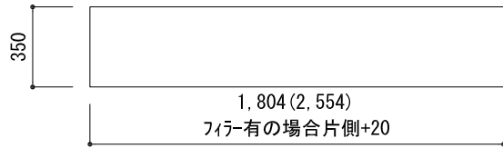
上面図
